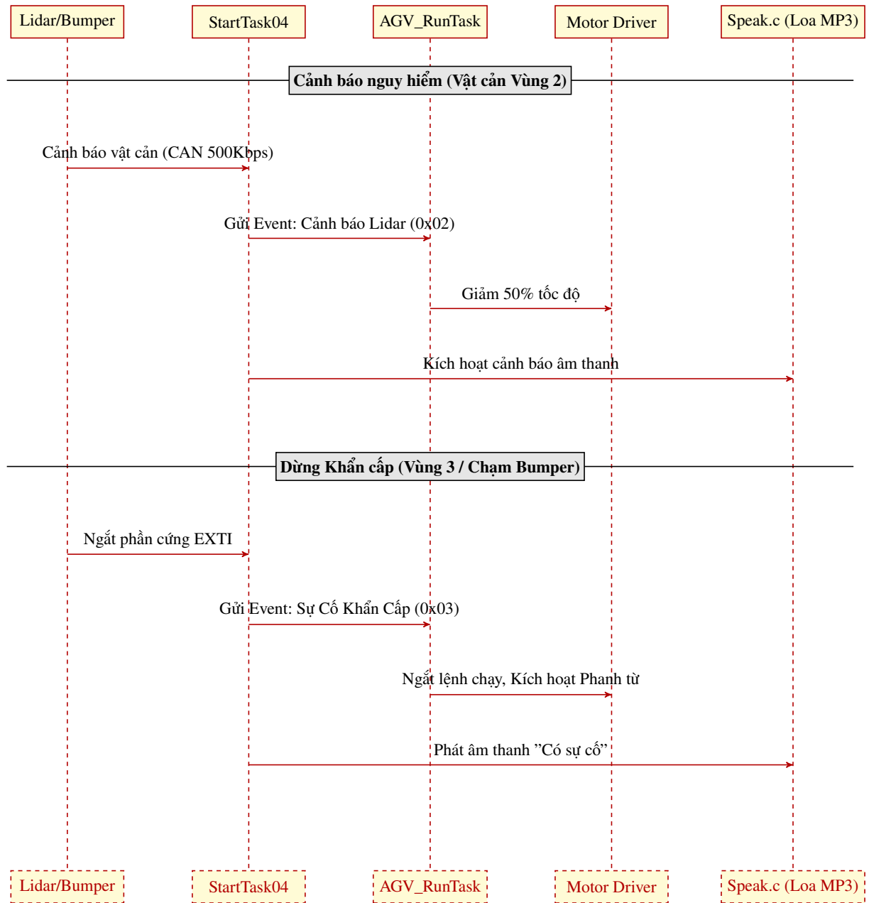
Hình 4.9 Sơ đồ tuần tự luồng giám sát an toàn và xử lý sự cố khẩn cấp.
