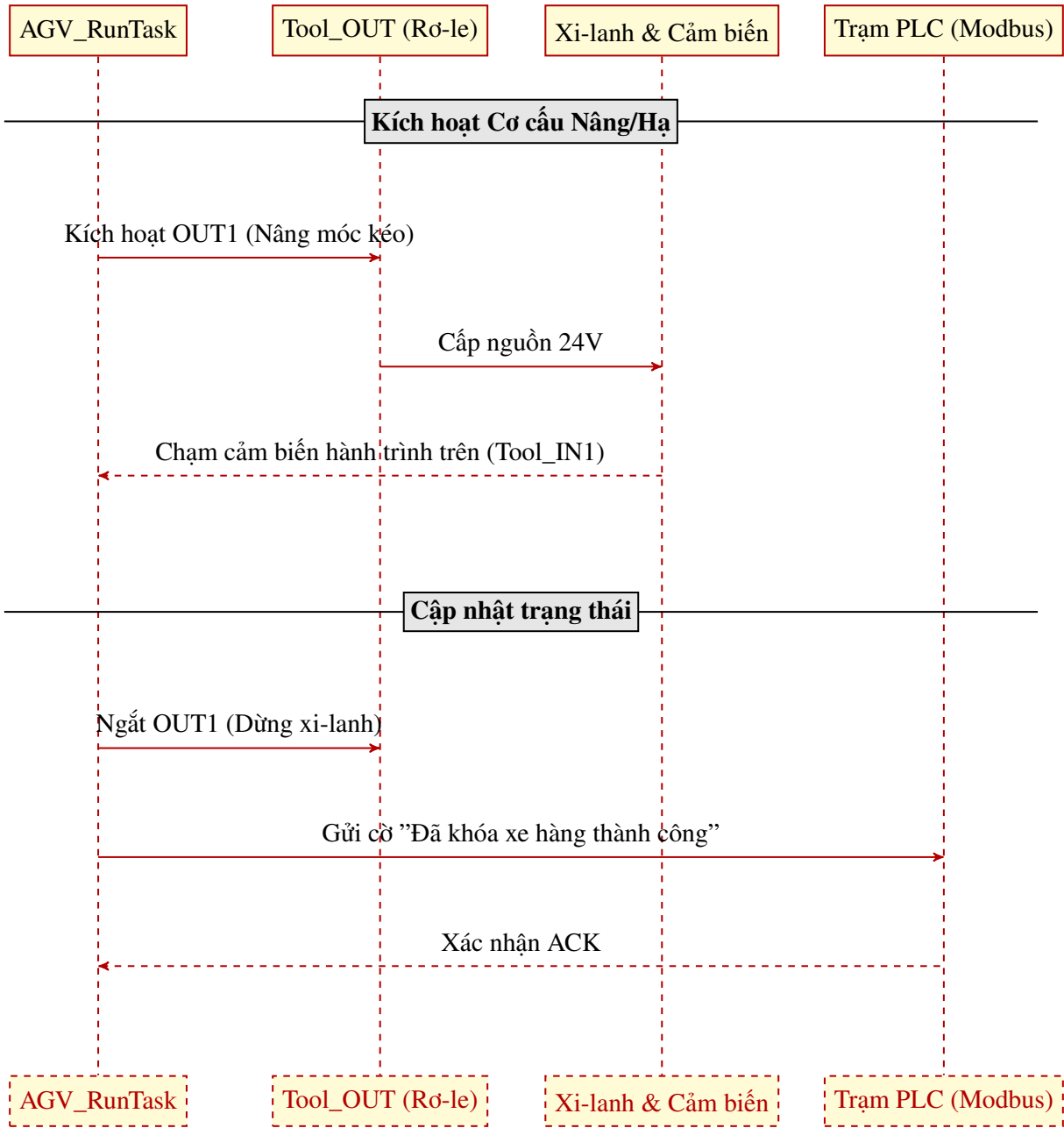
Hình 4.10 Sơ đồ tuần tự hoạt động của cơ cấu móc kéo xe hàng.
