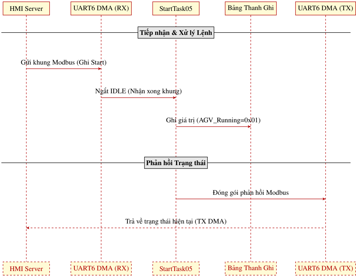
Hình 4.12 Sơ đồ tuần tự giao thức truyền thông Modbus RTU.
