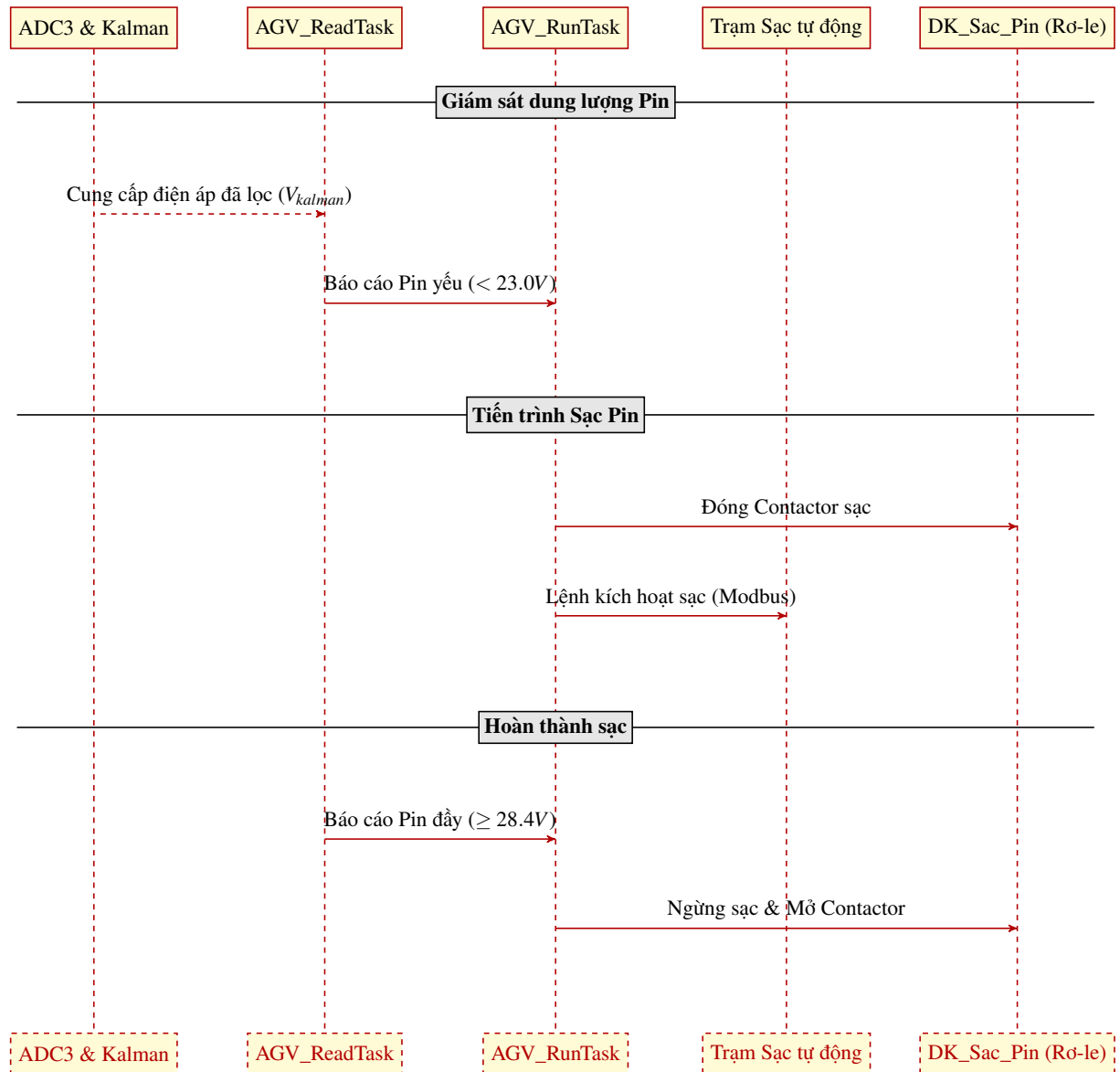
Hình 4.11 Sơ đồ tuần tự quá trình giám sát Pin và sạc tự động.
