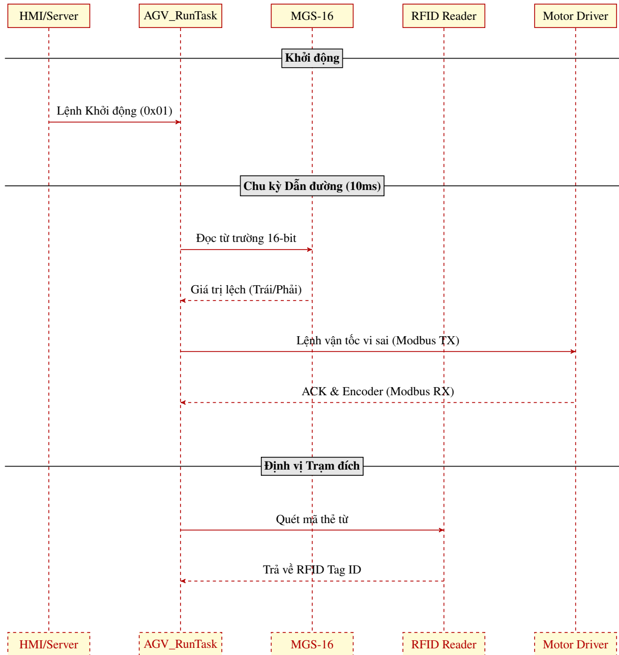
Hình 4.8 Sơ đồ tuần tự quá trình dẫn đường và nhận dạng trạm RFID.
